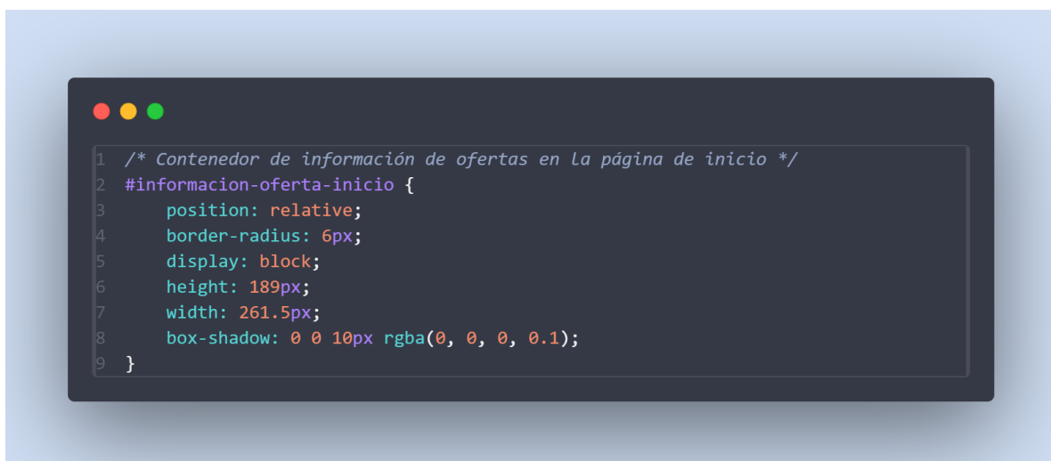
Figura 15 CSS Ofertitas en Inicio
