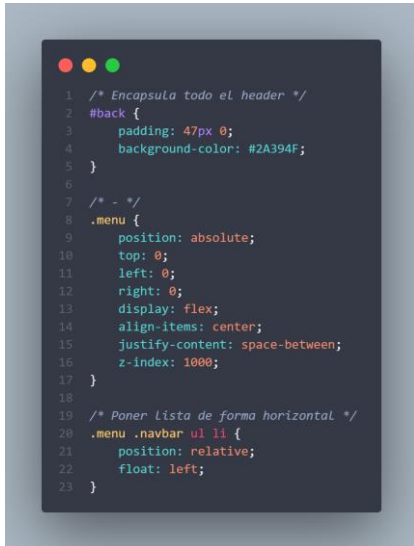
Figura 3 CSS del Header
